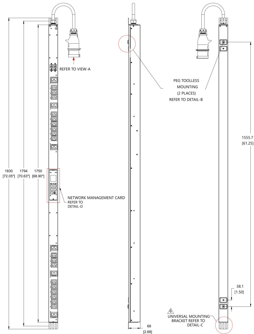
Рисунок 1 – Чертеж устройства
