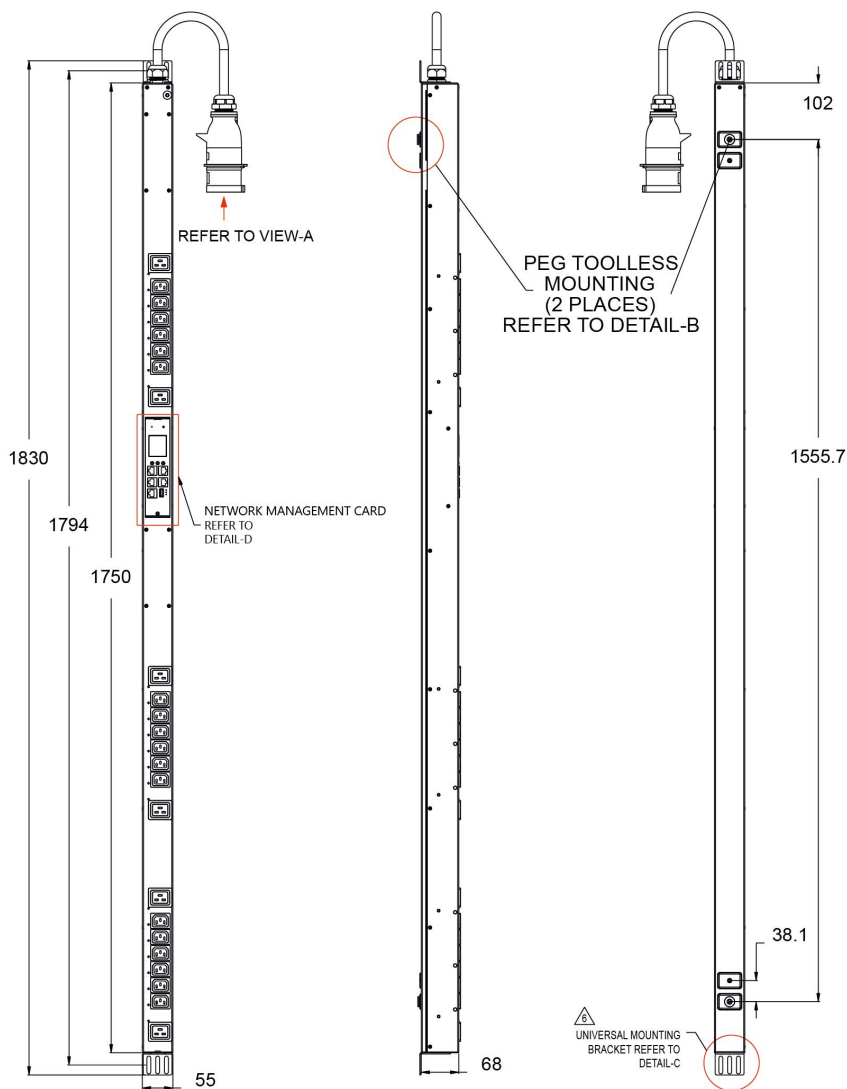
Рисунок 1 – Чертеж устройства
