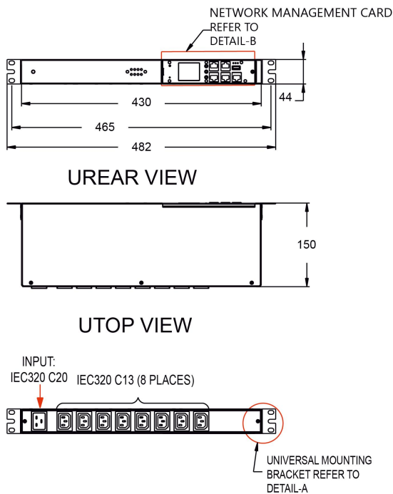
Рисунок 1 – Чертеж устройства
