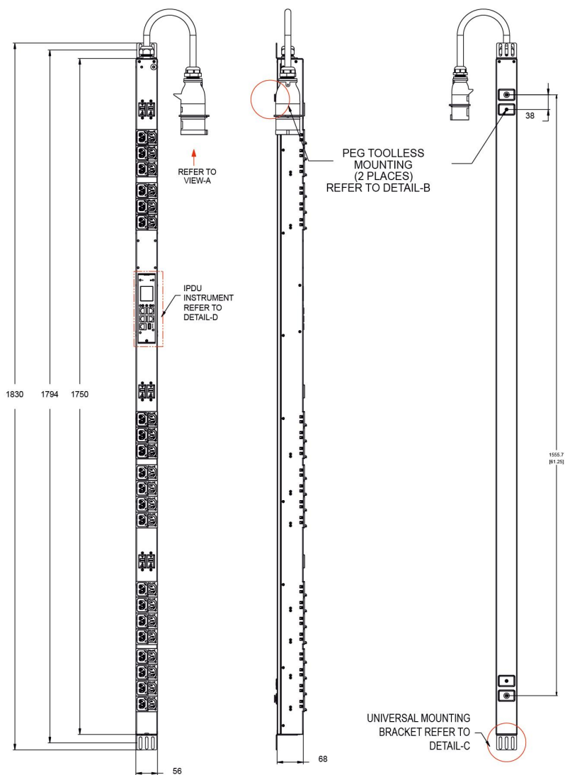
Рисунок 1 – Чертеж устройства
