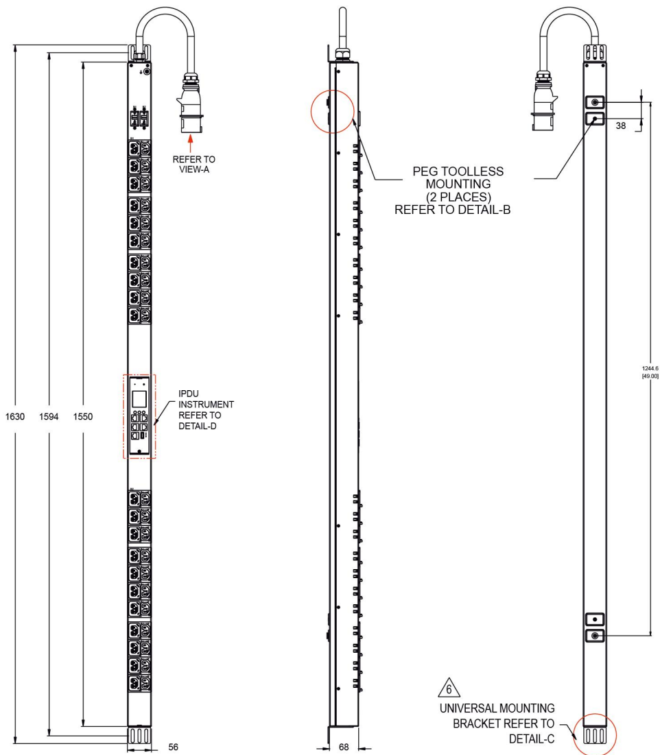
Рисунок 1 – Чертеж устройства
