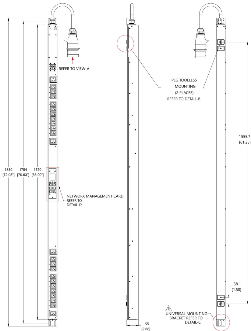
Рисунок 1 – Чертеж устройства
