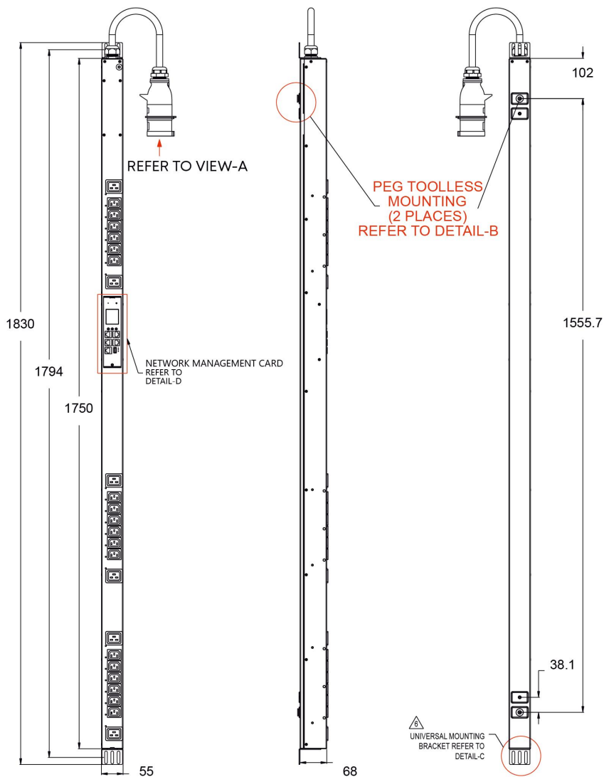
Рисунок 1 – Чертеж устройства
