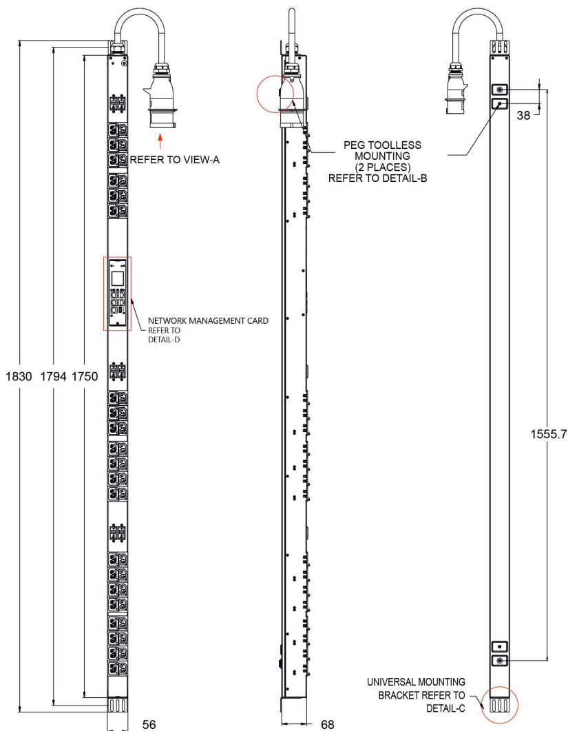
Рисунок 1 – Чертеж устройства
