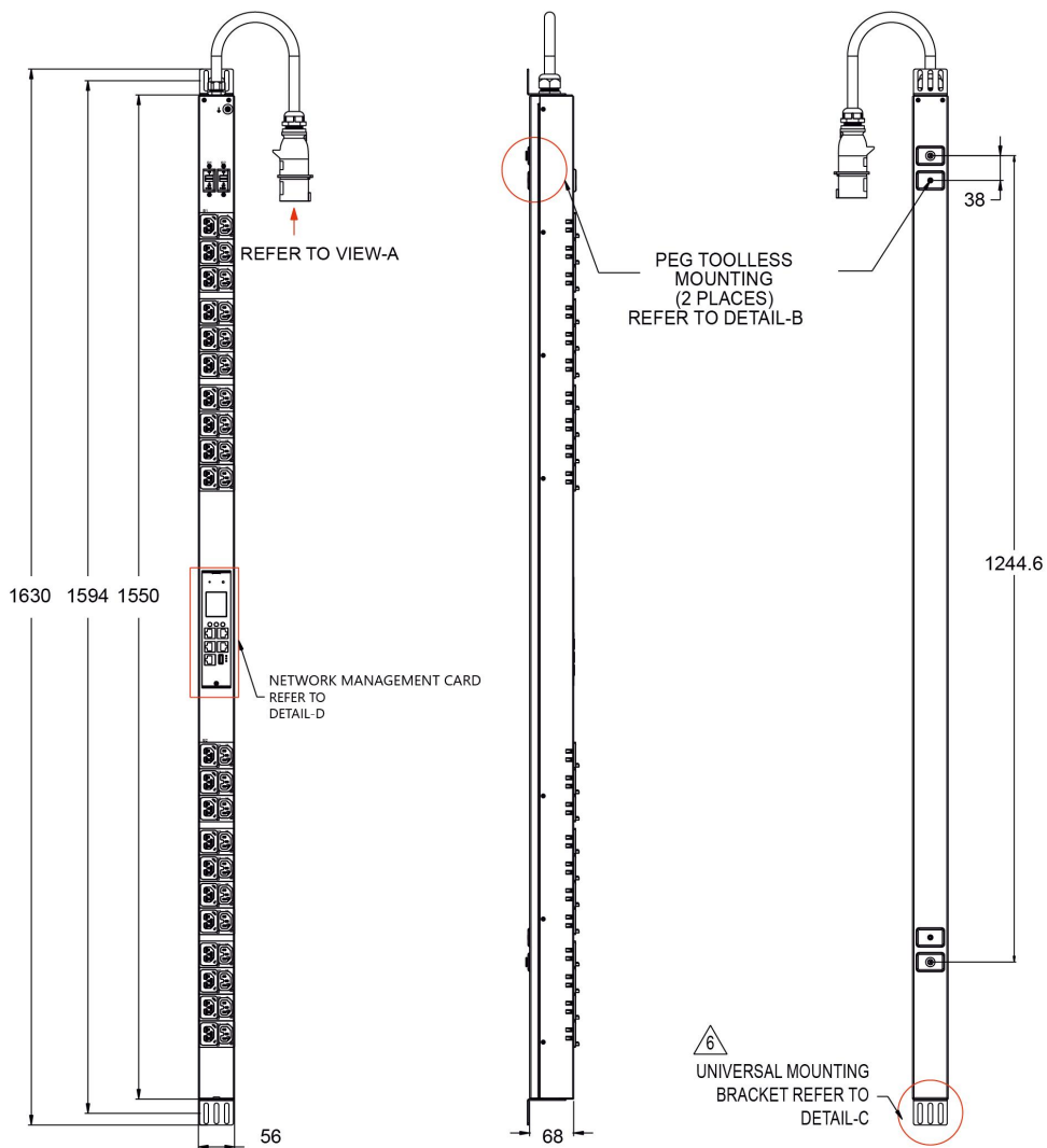
Рисунок 1 – Чертеж устройства
