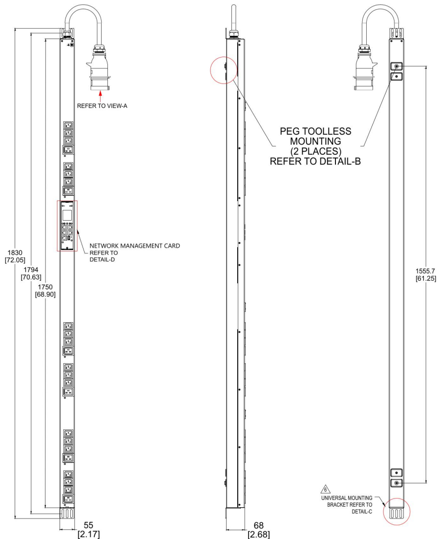
Рисунок 1 – Чертеж устройства
