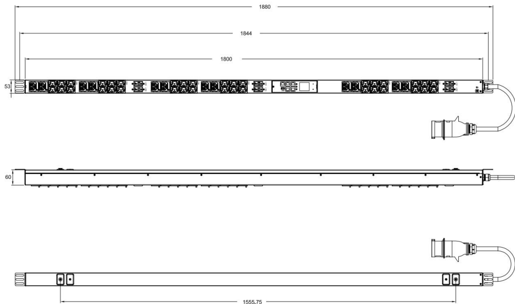
Рисунок 1 – Чертеж блока розеток SNR-PDU-A-36AL12ABL-32L3
