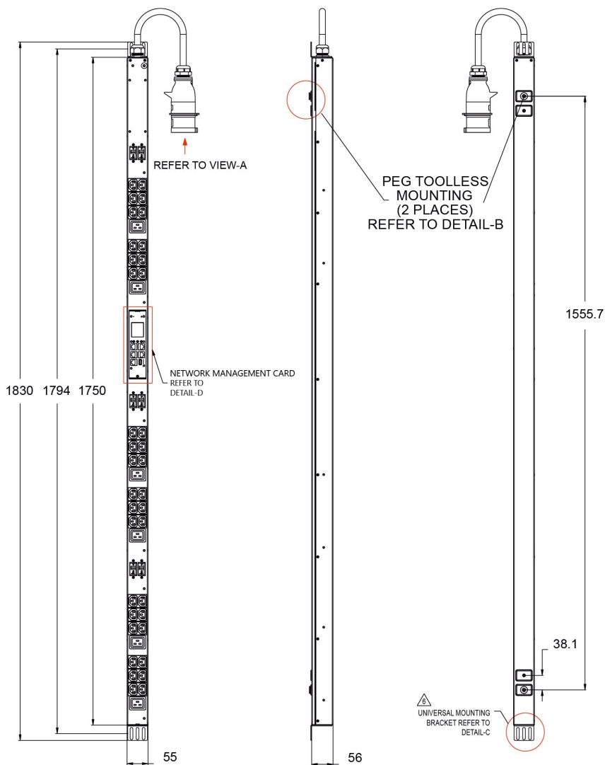
Рисунок 1 – Чертеж блока розеток SNR-PDU-A-36A06B-32L3
