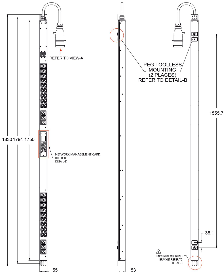
Рисунок 1 – Чертеж блока розеток SNR-PDU-A-36A06B-32L1
