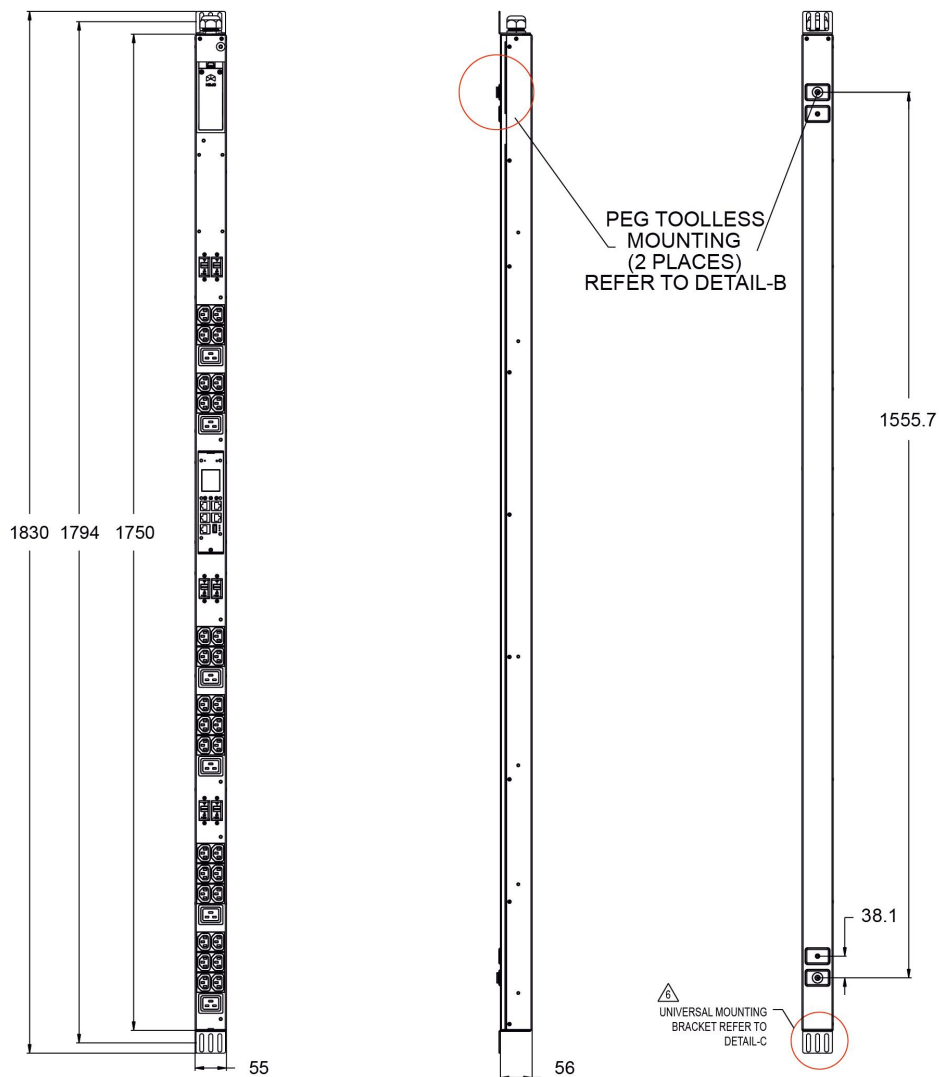
Рисунок 1 – Чертеж блока розеток SNR-PDU-A-30A06B-T32L3
