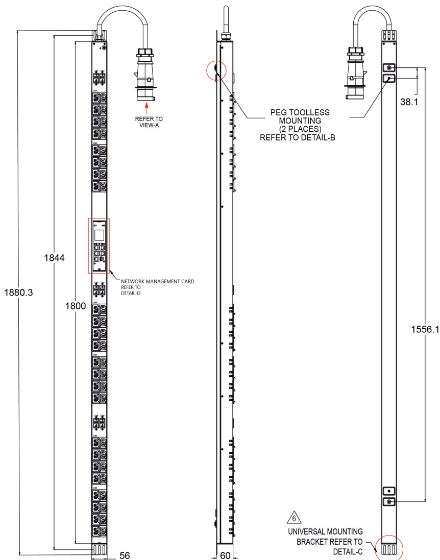
Рисунок 1 – Чертеж блока розеток SNR-PDU-A-24AL24ABL-32L3
