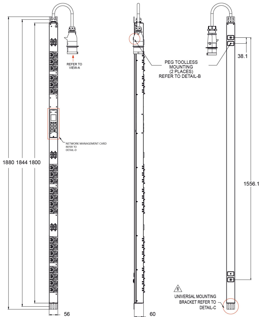
Рисунок 1 – Чертеж блока розеток SNR-PDU-A-21AL21ABL-32L3
