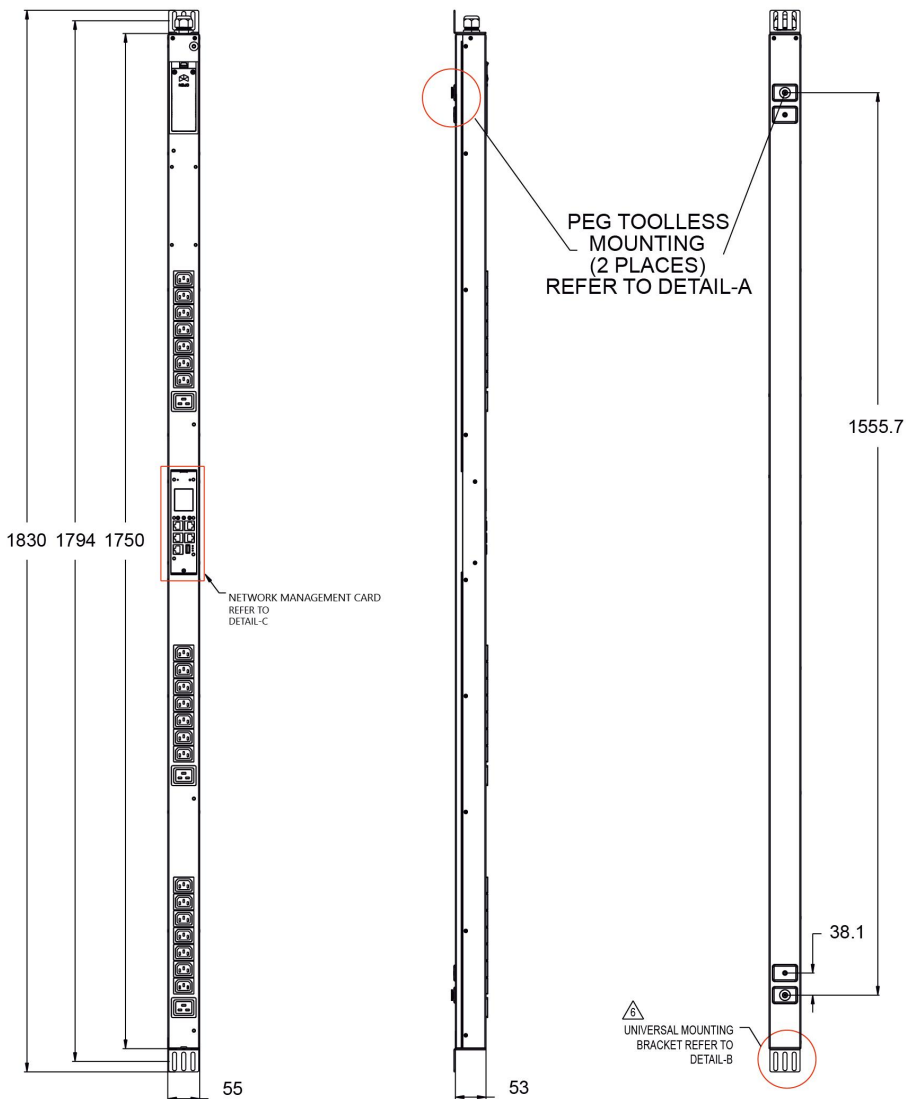
Рисунок 1 – Чертеж блока розеток SNR-PDU-A-21A03B-T16L3
