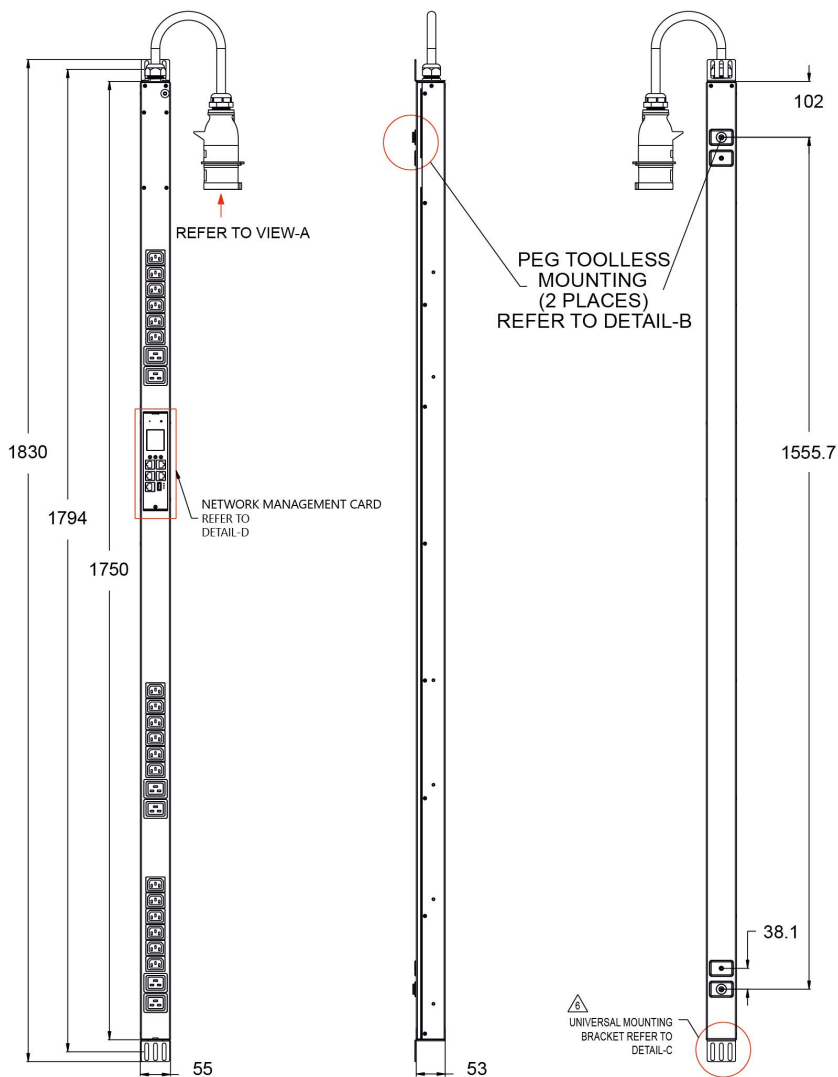
Рисунок 1 – Чертеж блока розеток SNR-PDU-A-18A06B-16L3
