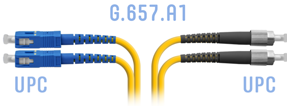
Рисунок 1 - Общий вид
