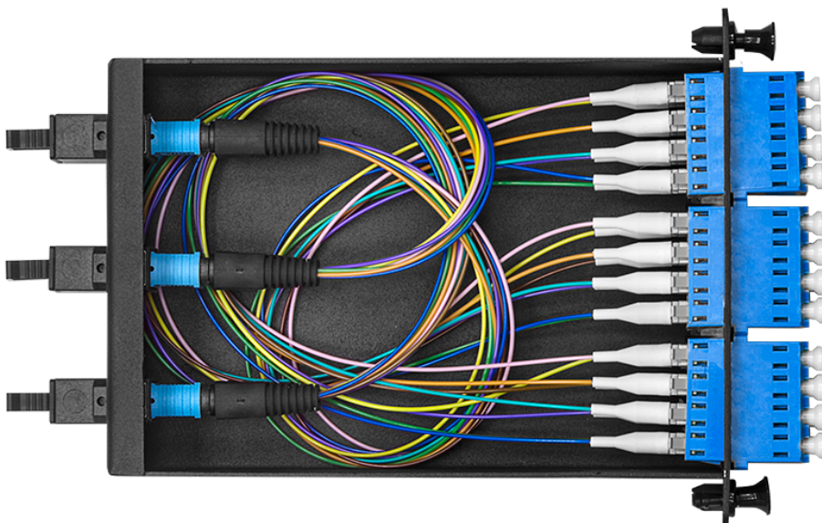
Рисунок 2 - Внутренний конструктив
