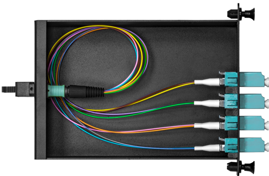
Рисунок 2 - Внутренний конструктив
