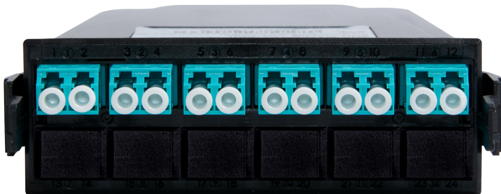
Рисунок 1 - Общий вид
