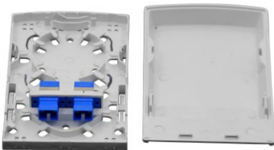
Рисунок 2 - Внутренний конструктив
