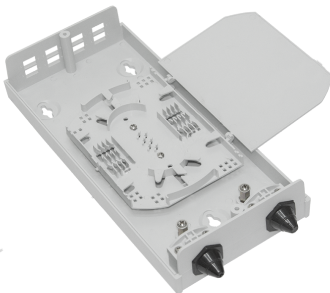
Рисунок 2 - Внутренний конструктив
