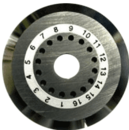
Рисунок 1 - Общий вид
