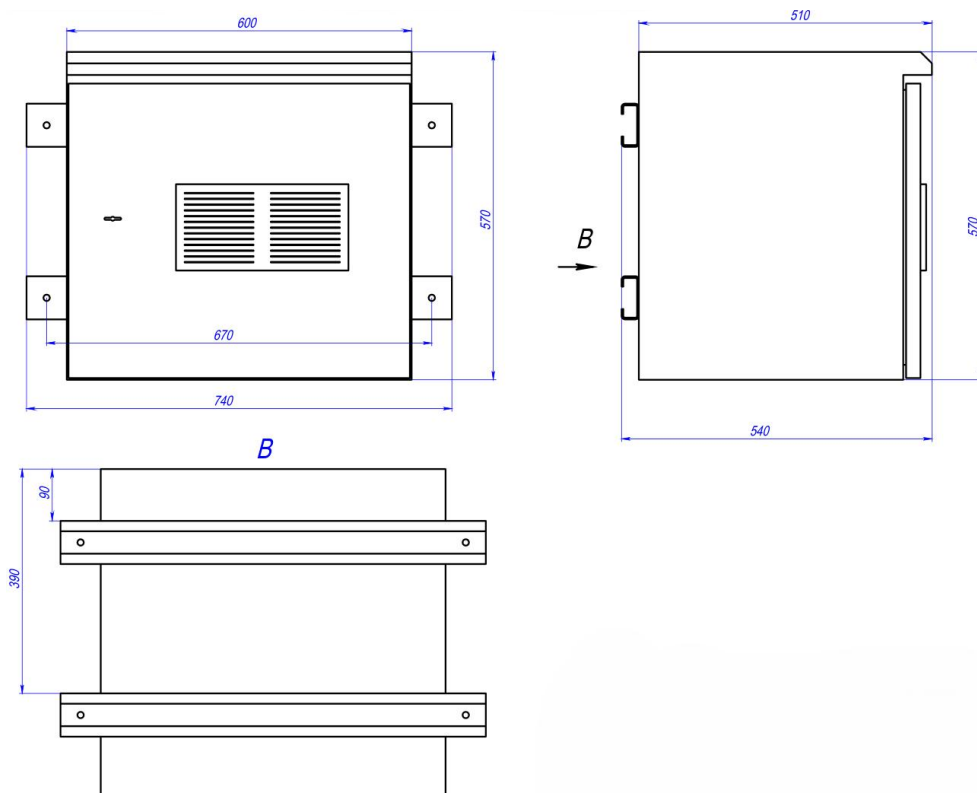
Рисунок 2 – Габаритные размеры
