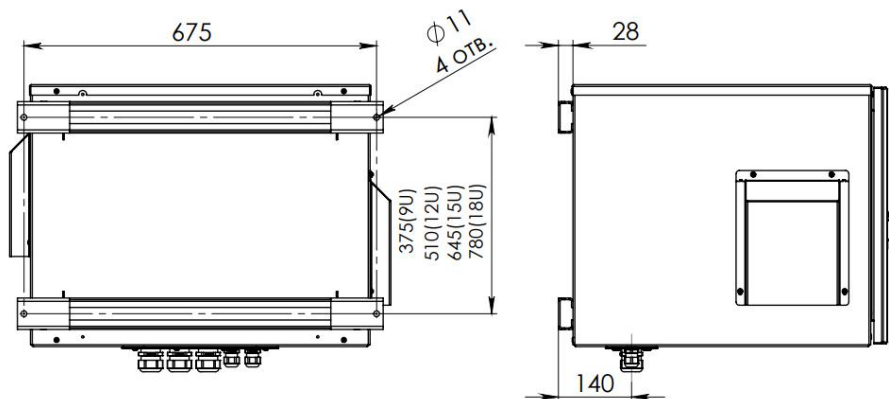
Рисунок 5 - Установка на столб
