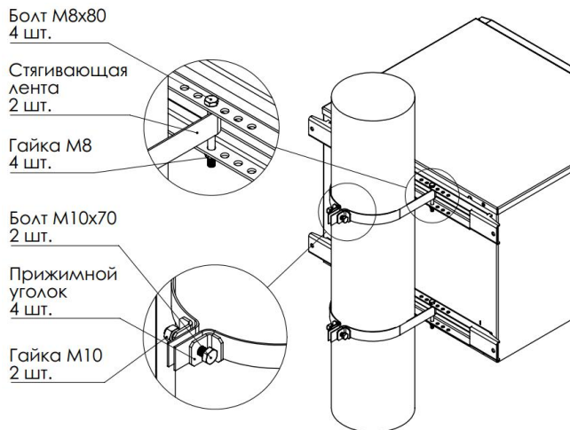
Рисунок 5 - Установка на столб
