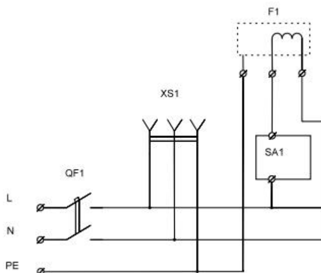
Рисунок 8 - Схема электрическая принципиальная
