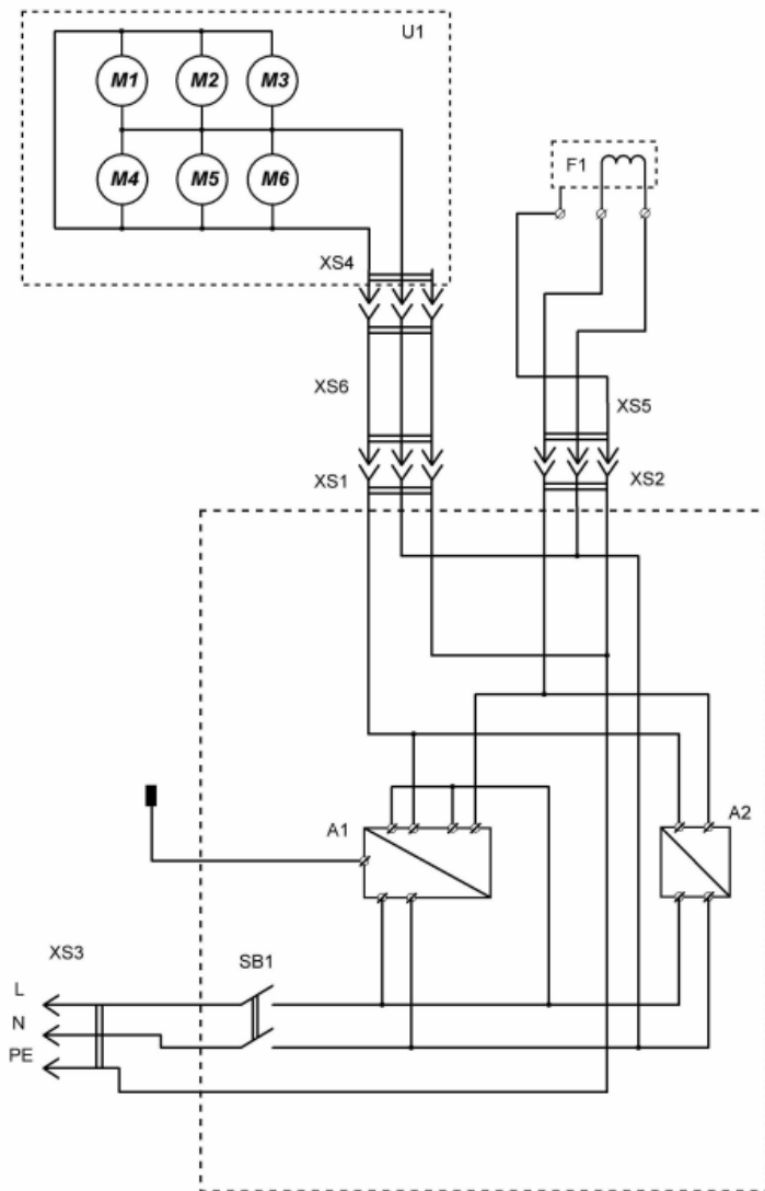
РИСУНОК 4 – СХЕМА ЭЛЕКТРИЧЕСКАЯ ПРИНЦИПИАЛЬНАЯ
