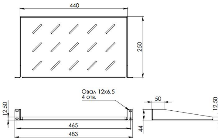
Рисунок 3 – Габаритные размеры
