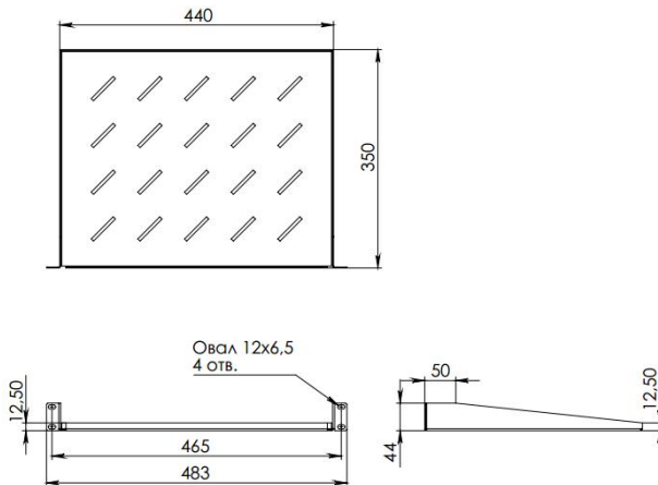
Рисунок 3 – Габаритные размеры
