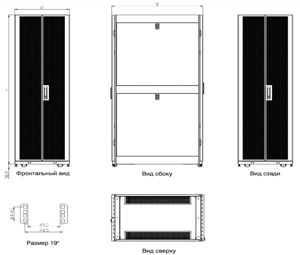
Рисунок 3 - Габаритные размеры шкафа
