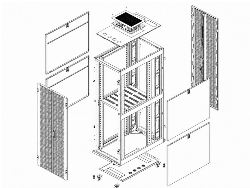
Рисунок 1 – Комплектация шкафа
