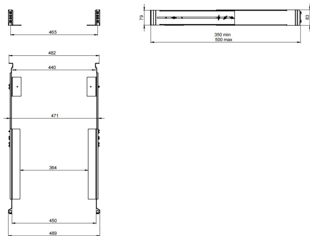
Рисунок 1 – Чертёж салазок
