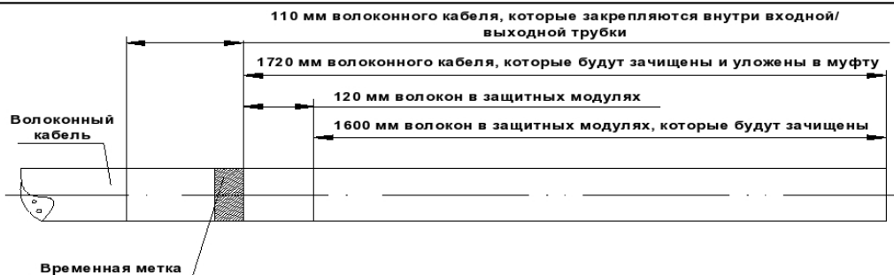
Рисунок 5.2 - Определение длины волоконного кабеля
