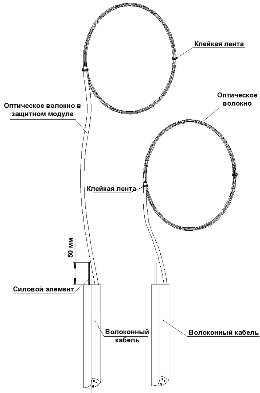
Рисунок 5.4 - Разделение оптических волокон
