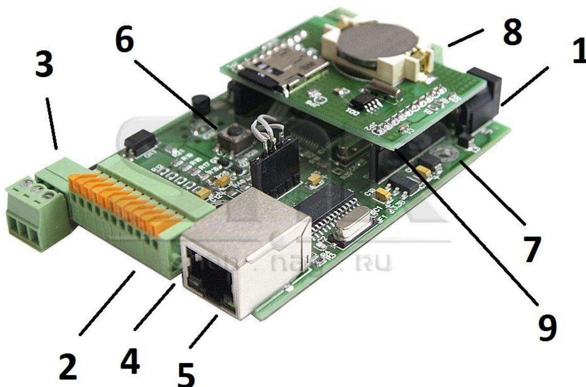
Рисунок 2 – Контакты и рабочие узлы устройства
