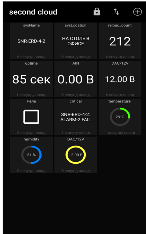
Рисунок 17 – Пример итоговой конфигурации
