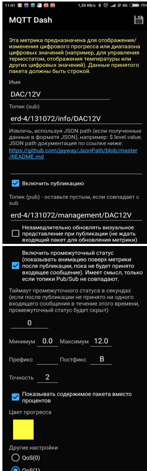
Рисунок 15 – Пример конфигурации метрики диапазон, позволяющей отображать и изменять состояние выхода DAC/12V устройства
