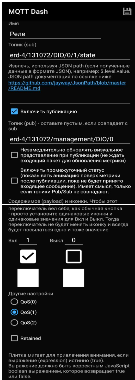
Рисунок 14 – Пример конфигурации метрики переключатель, позволяющей отображать и изменять состояние реле устройства
