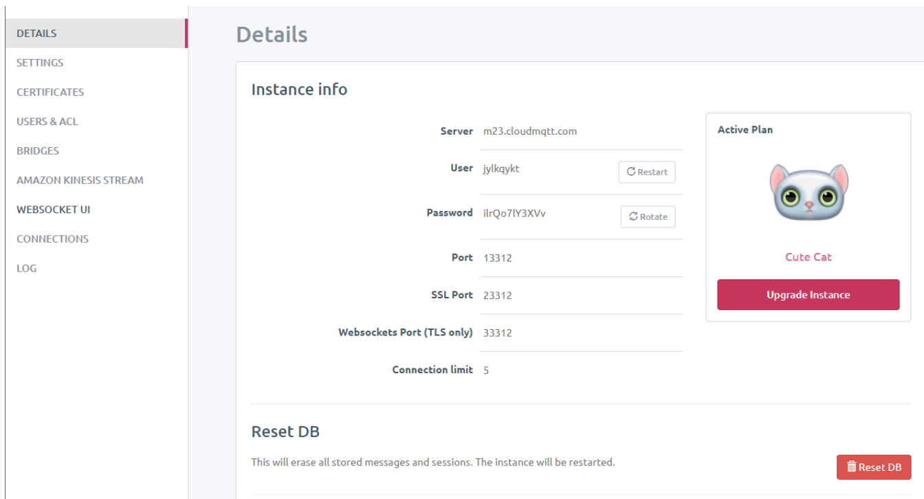
Рисунок 3 – Основные реквизиты брокера
