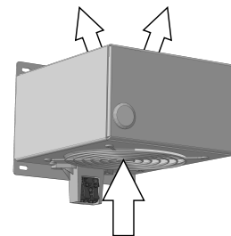
Рисунок 1. Рекомендованное монтажное положение
