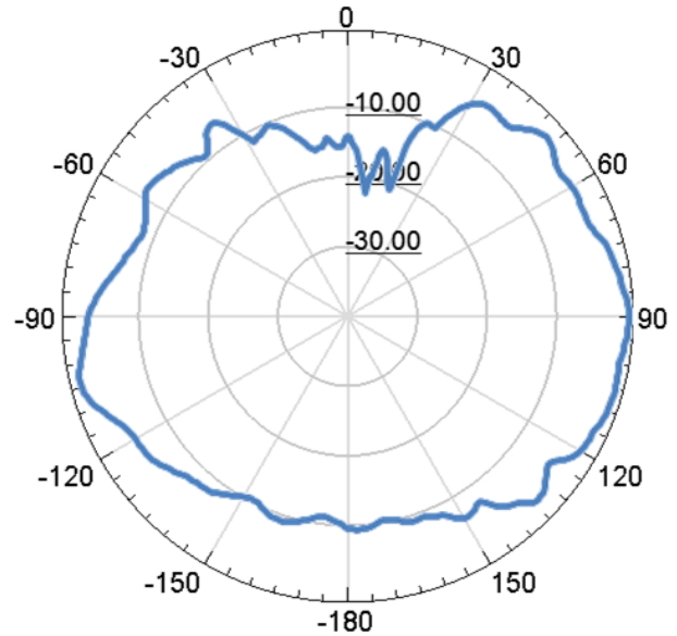
5GHz (Vertical)
