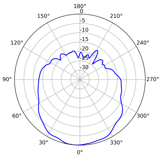
5GHz (Horizontal)
