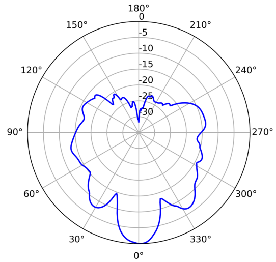
6GHz (Vertical)
