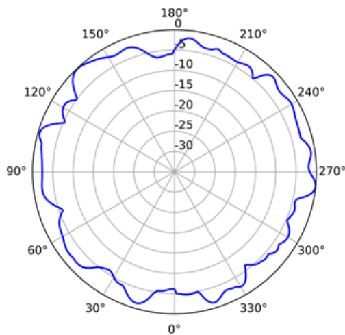
6GHz (Horizontal)
