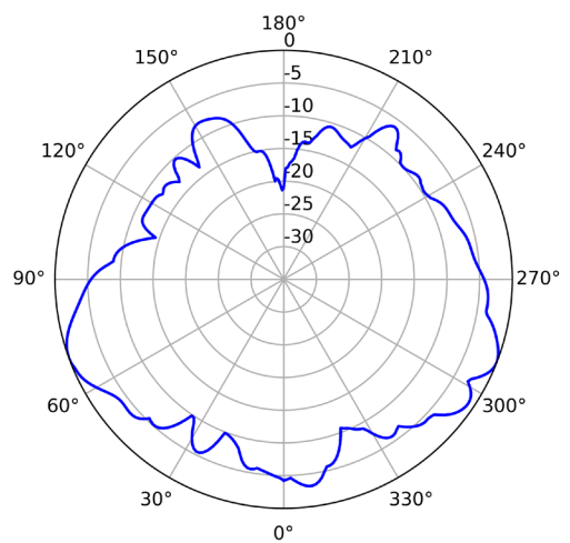
6GHz (Vertical)
