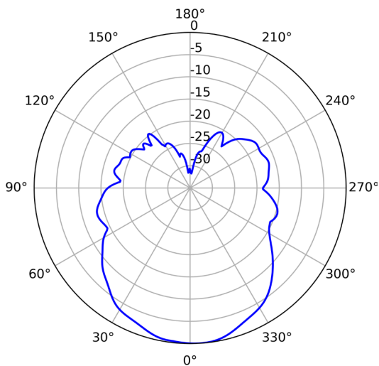
6GHz (Horizontal)
