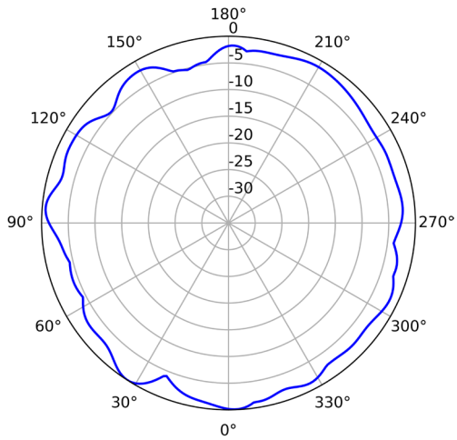
5GHz (Horizontal)
