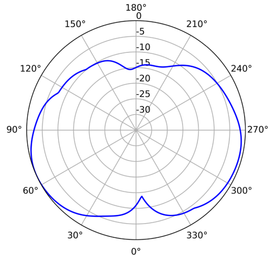
2.4GHz (Vertical)
