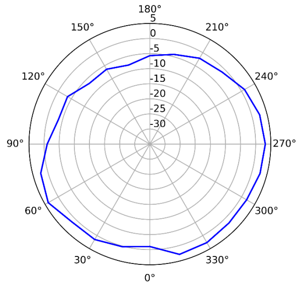
5GHz (Vertical)
