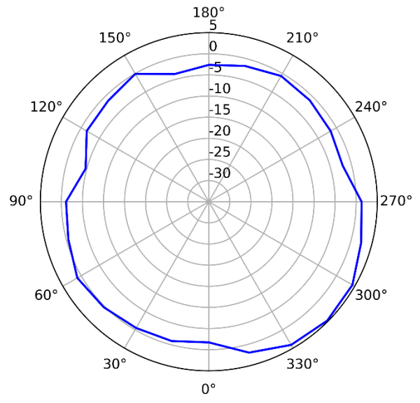
2.4GHz (Vertical)
