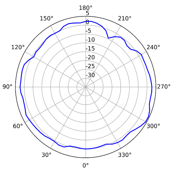
5GHz (Horizontal)
