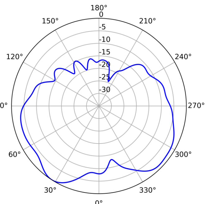
5GHz (Vertical)
