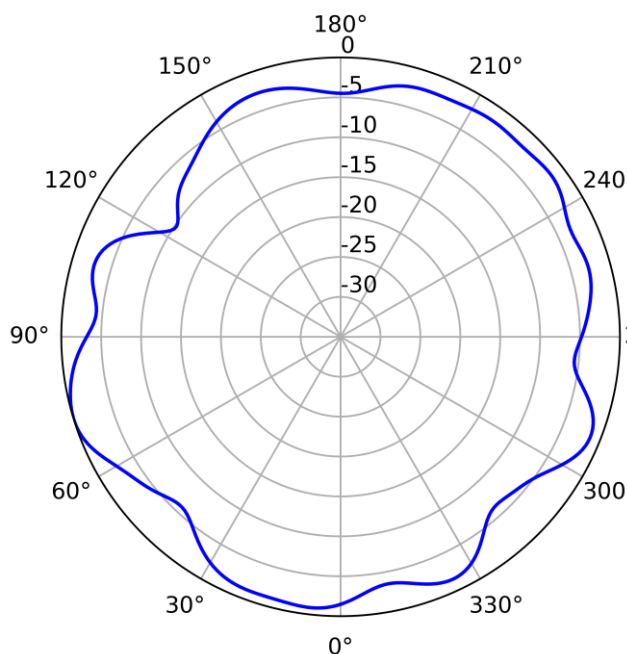
5GHz (Horizontal)
