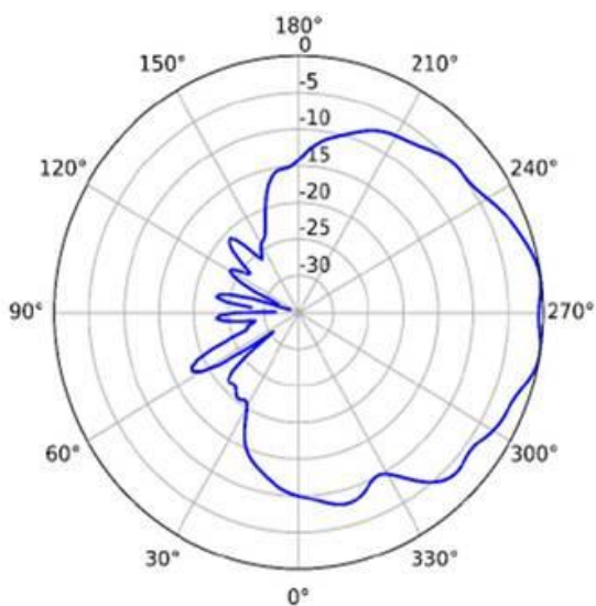
5GHz (Horizontal)
