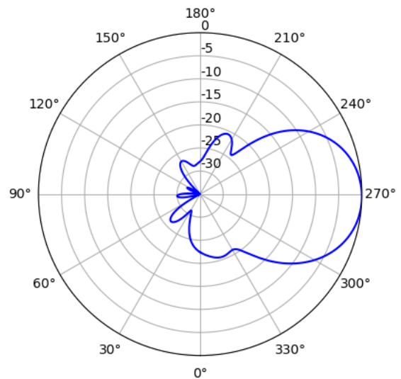
2.4GHz (Vertical)
