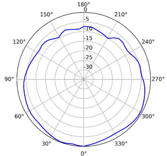
2.4GHz (Vertical)
