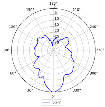
5GHz (Vertical)
