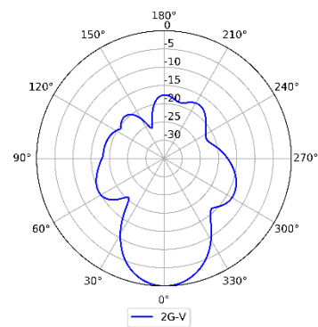
2.4GHz (Vertical)
