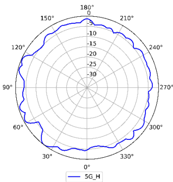
5GHz (Horizontal)
