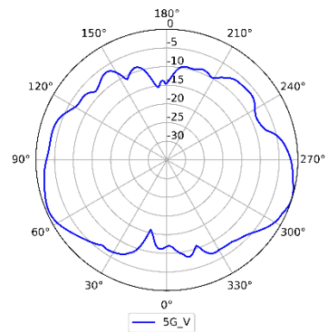
5GHz (Vertical)
