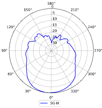
5GHz (Horizontal)
