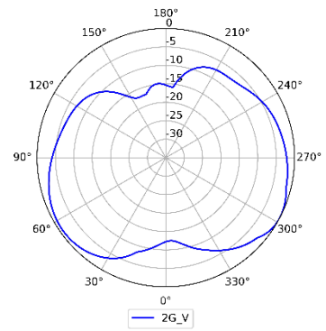
2.4GHz (Vertical)
