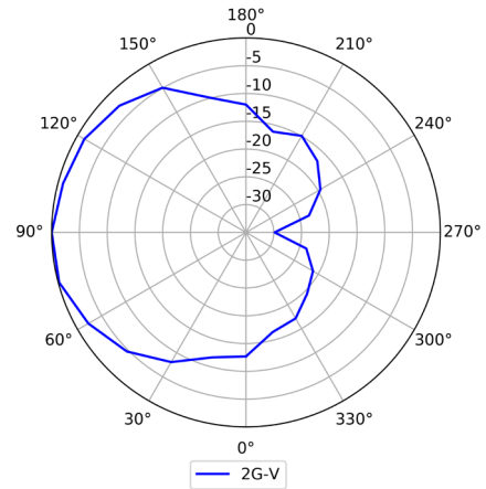
2.4GHz (Vertical)
