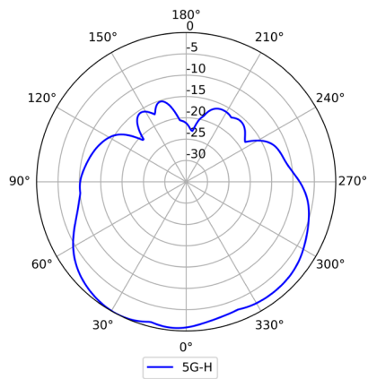
5GHz (Horizontal)
