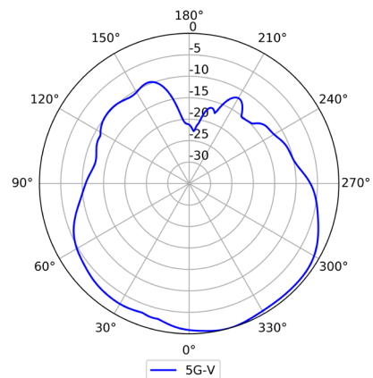
5GHz (Vertical)
