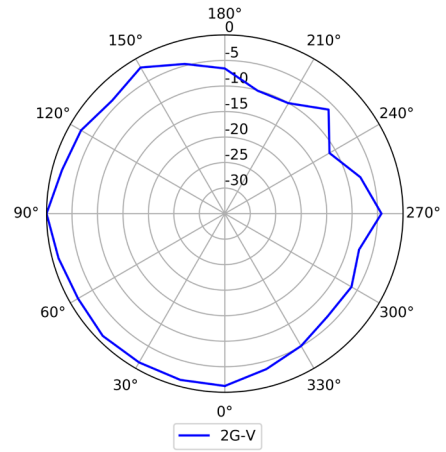
2.4GHz (Vertical)
