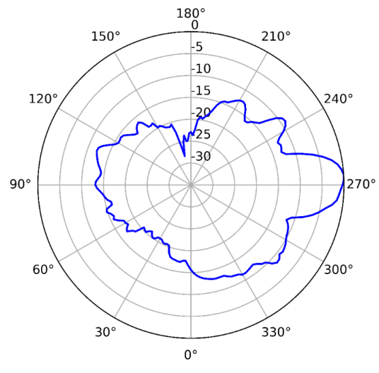
5GHz (Vertical)
