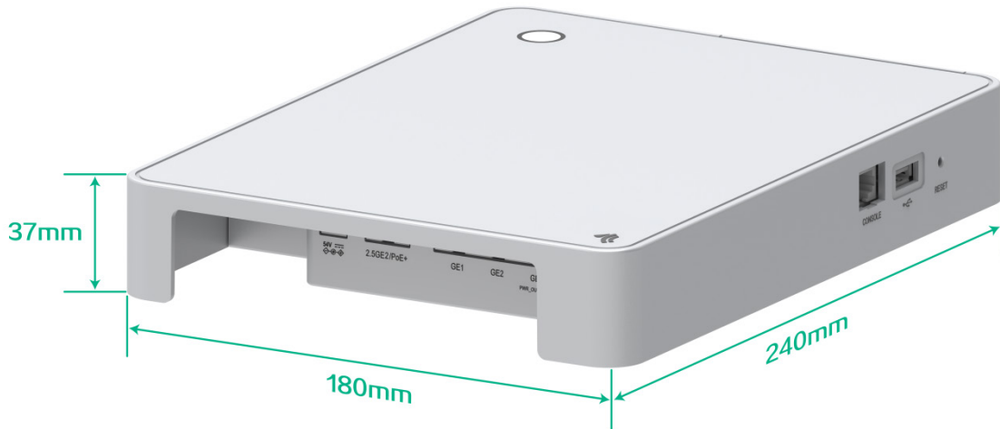
图2-30 设备尺寸图
