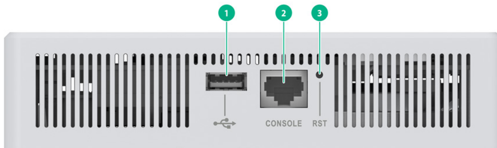
图2-16 设备接口示意图 3
