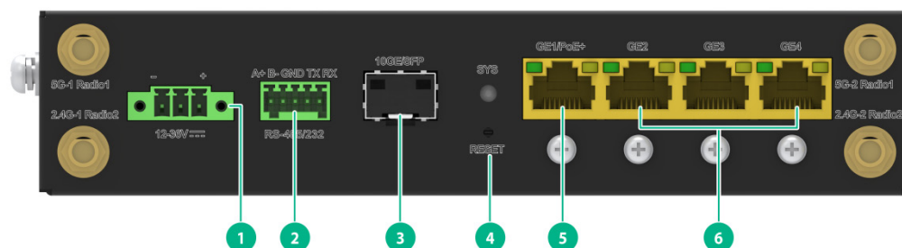
图2-7 接口示意图
