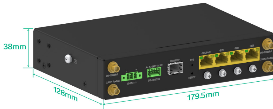
图2-6 设备尺寸图
