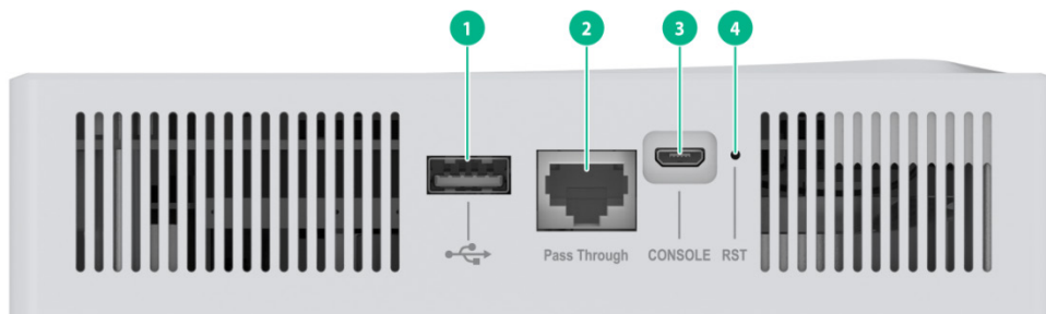
图2-21 设备接口示意图 3
