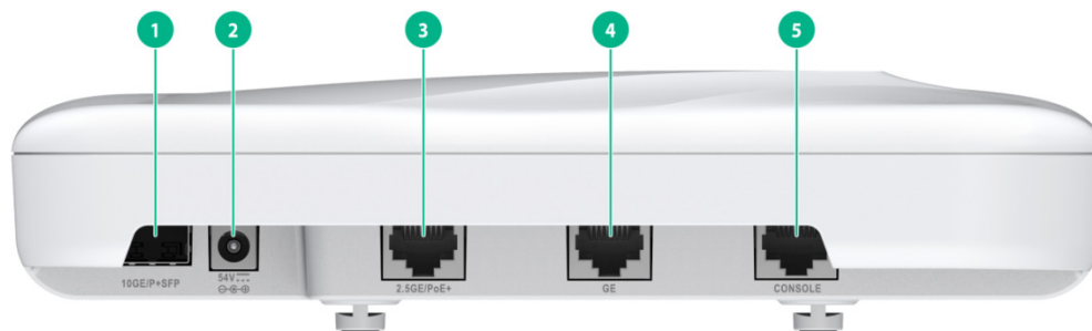
图2-35 接口示意图 1
