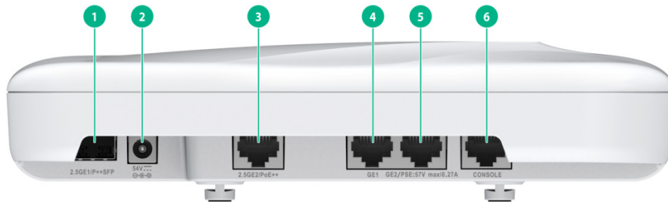
图2-45 接口示意图 1
