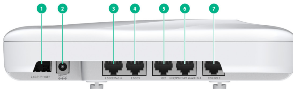
图2-40 接口示意图 1
