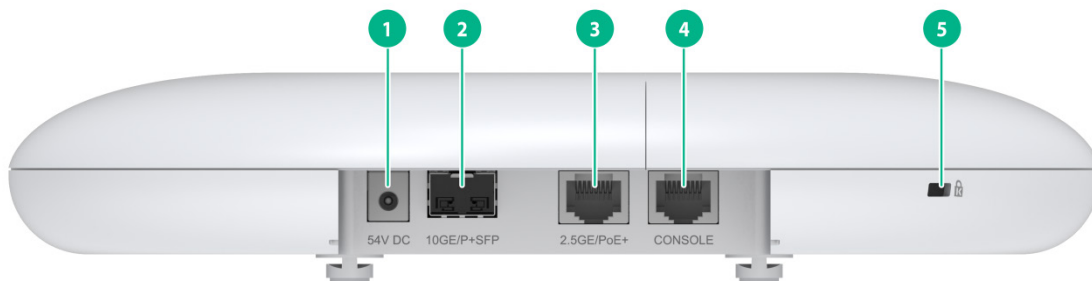
图2-50 接口示意图 1
