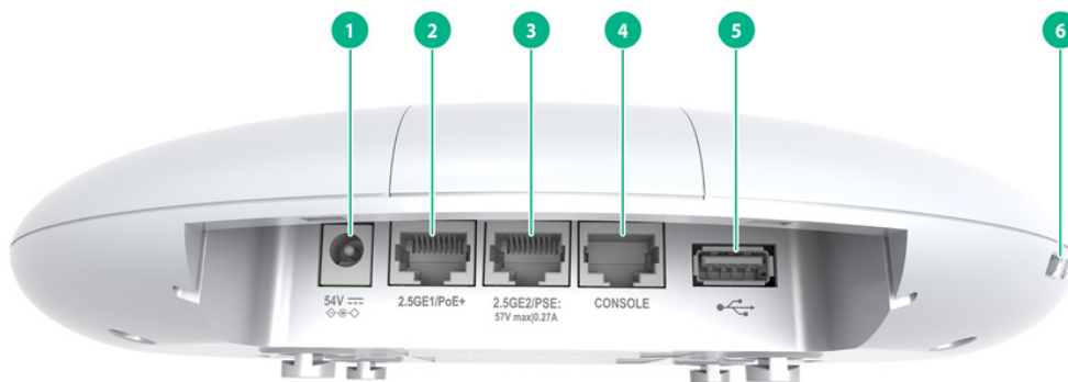
图2-24 接口示意图 1
