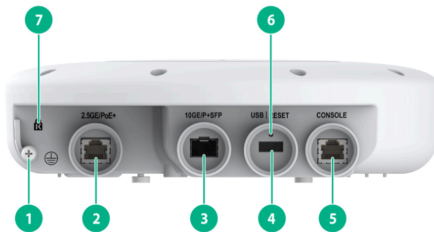
图2-28 接口示意图
