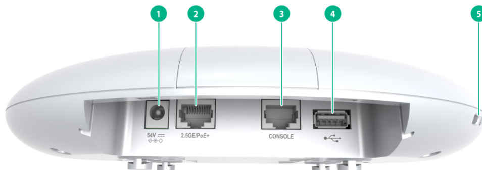
图2-3 接口示意图 1
