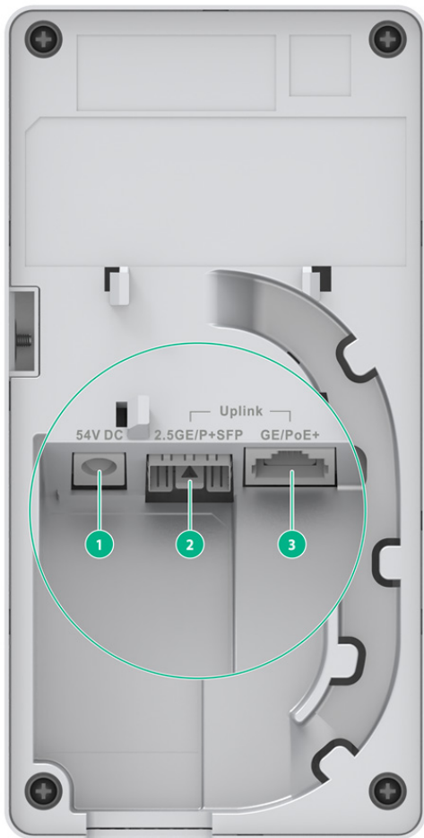
图2-15 接口示意图 2
