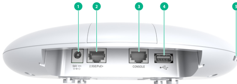
图2-10 接口示意图 1
