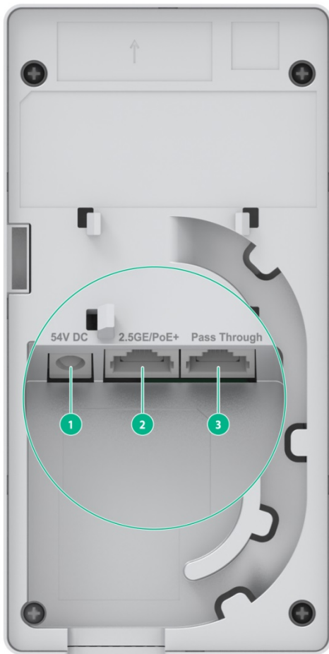
图2-20 接口示意图 2
