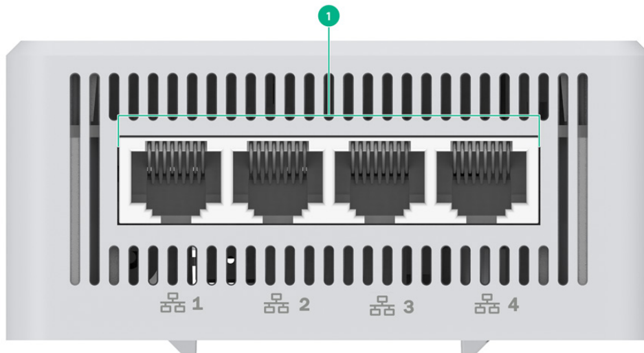
图2-14 接口示意图 1
