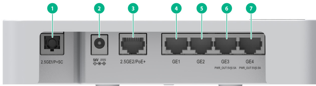
图2-31 接口示意图 1
