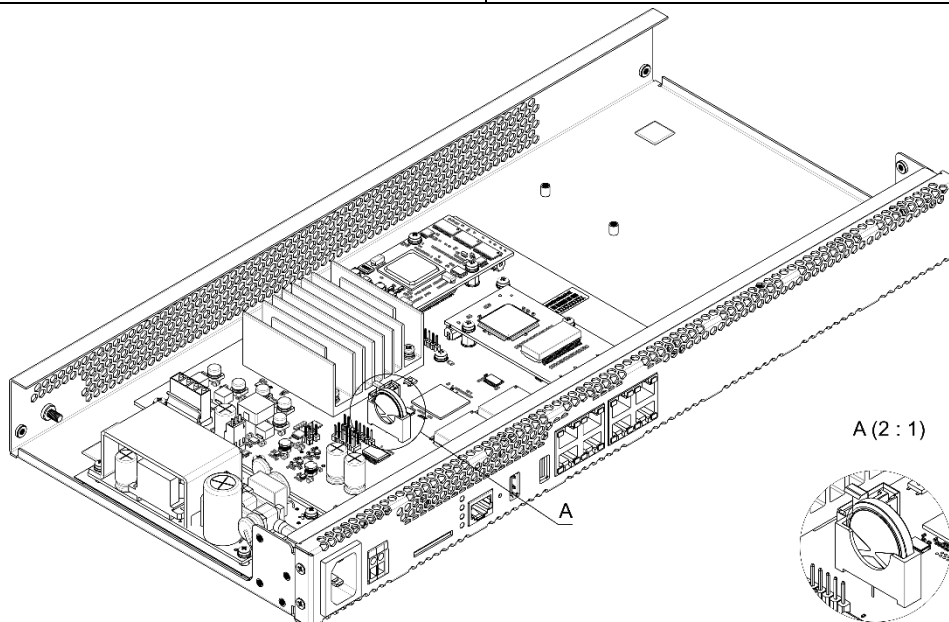
Рисунок 15 – Положение батарейки RTC
