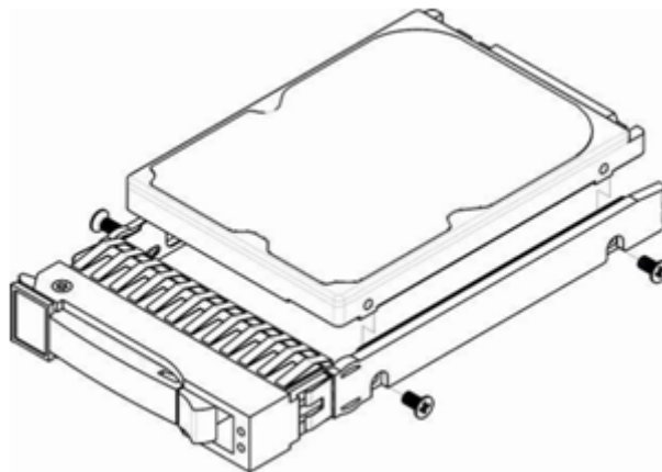
Рисунок 40 – Крепление SATA-диска в лоток направляющих салазок
