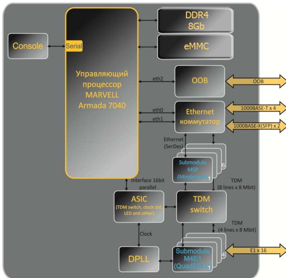
Рисунок 11 – Функциональная схема SMG-3016
