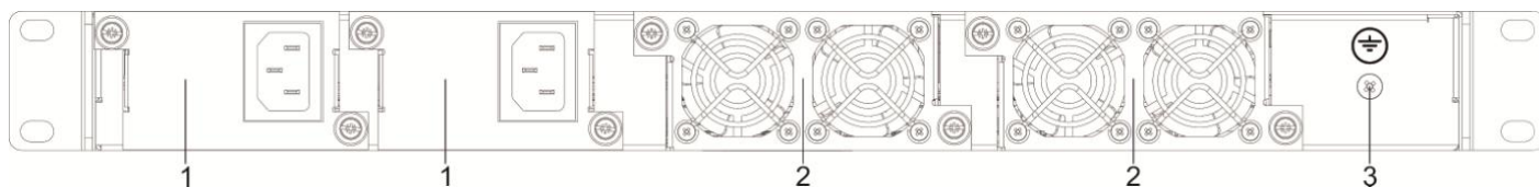
Рисунок 18 – Внешний вид задней панели SMG-3016
