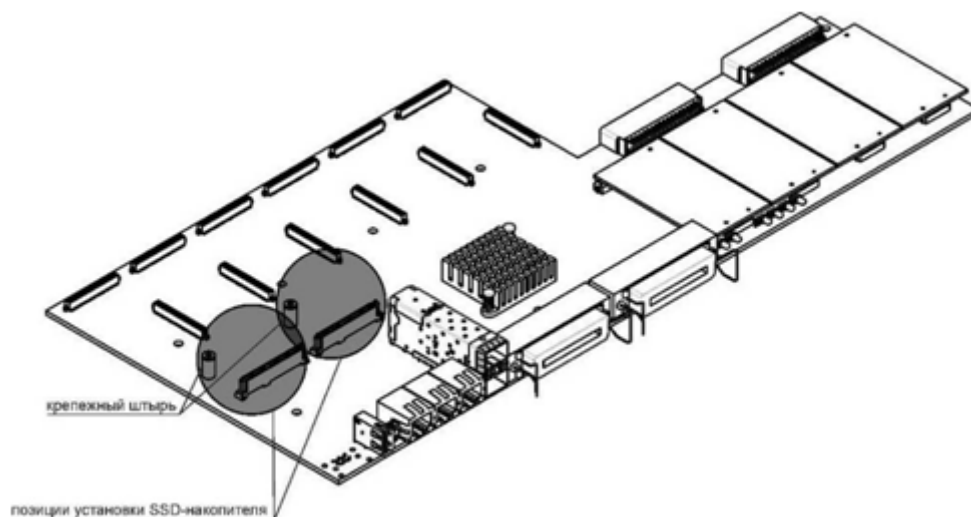
Рисунок 37 – Установка SSD-накопителя
