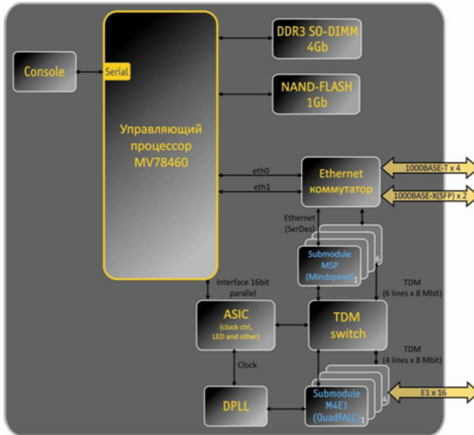
Рисунок 10 – Функциональная схема SMG-2016
