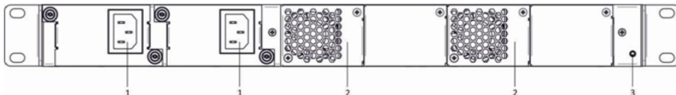
Рисунок 14 – Внешний вид задней панели SMG-1016M
