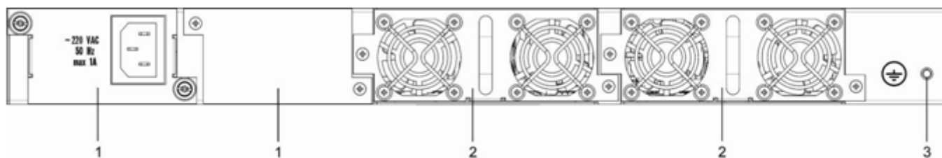
Рисунок 16 – Внешний вид задней панели SMG-2016
