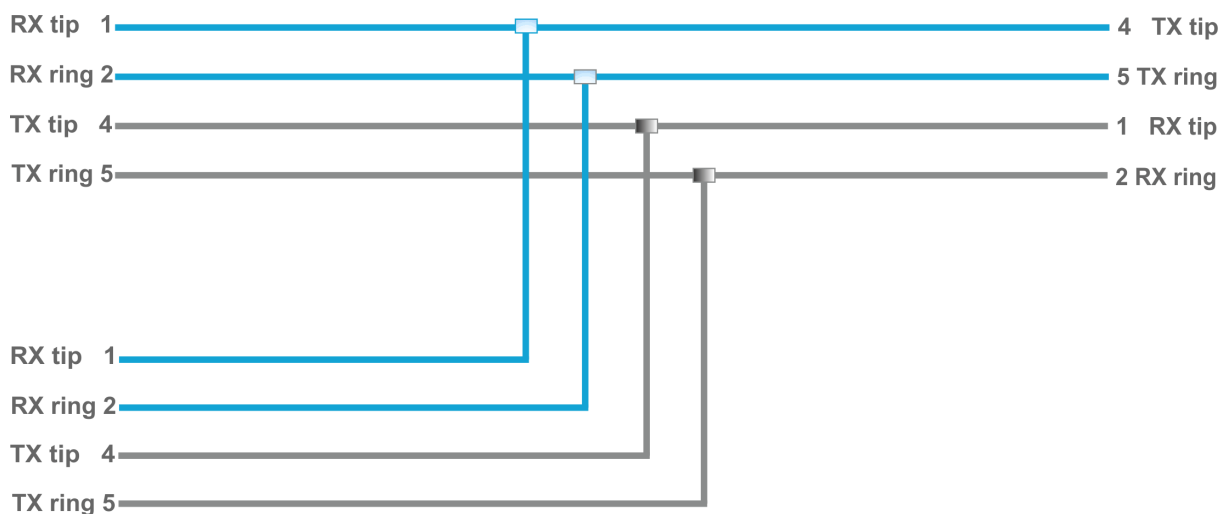
Схема распайки кабеля для резервирования E1
