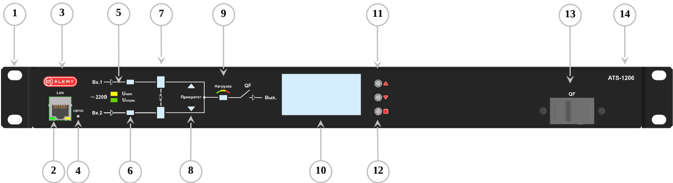
Рисунок 1 – Электронно-механический АСП ATS-1206 , передняя панель:
